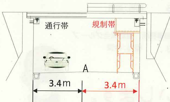
●規制イメージ図（片側交互通行規制） 市道 三ヶ日都筑丸田線、工事中
