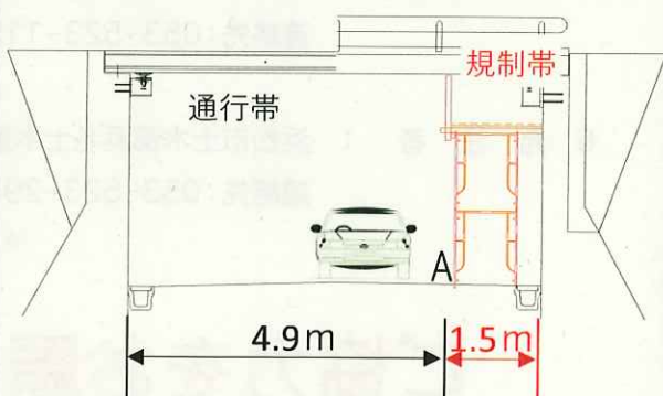
●規制イメージ図（路肩規制） 市道 三ヶ日都筑丸田線、工事時間外
